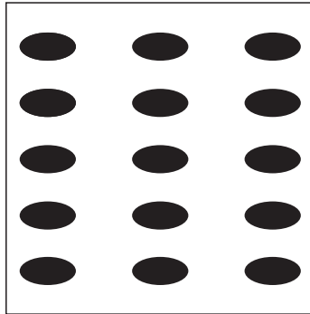
OS minta: 8x16 mm kiosztás: függőleges tengelytáv: 30 mm nyitott felület: ~10%
