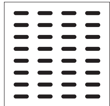
O330-20 V minta: 5x19 mm kiosztás: függőleges tengelytáv: 30-20 mm nyitott felület: ~15%
