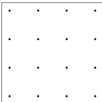
K340 minta: 3 mm Ø kiosztás: függőleges tengelytáv: 40 mm nyitott felület: ~0,4%
