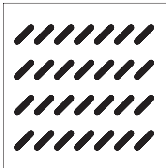
O330-20 D minta: 5x19 mm kiosztás: függőleges tengelytáv: 30-20 mm nyitott felület: ~15%
