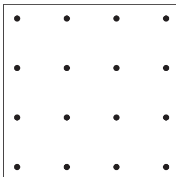
K540 minta: 5 mm Ø kiosztás: függőleges tengelytáv: 40 mm nyitott felület: ~1%
