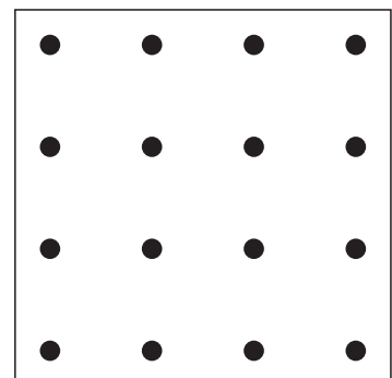
K840 minta: 8 mm Ø kiosztás: vízszintes tengelytáv: 40 mm nyitott felület: ~3%
