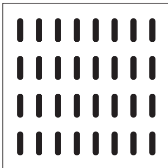
O330-20 F minta: 5x19 mm kiosztás: függőleges tengelytáv: 30-20 mm nyitott felület: ~15%
