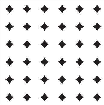
RQ 825 F minta: 8x8 mm kiosztás: függőleges tengelytáv: 25 mm nyitott felület: ~8%
